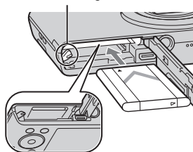
Akumulatora izgrūšanas svira
